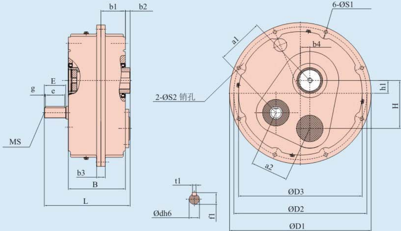
SLXG35-SLXG125 的外形尺寸 SLXG35- SLXG125 Dimensions
