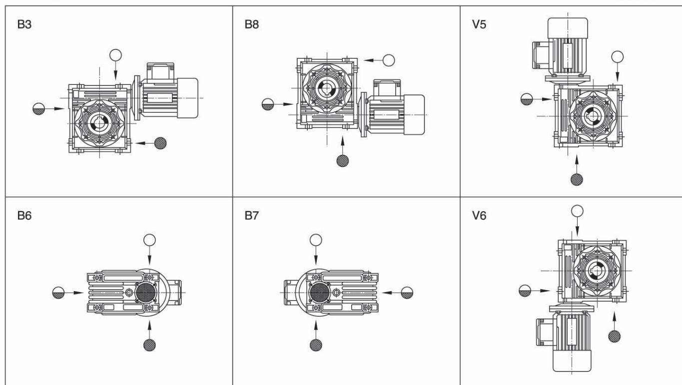
安装型式 Mounting positions
